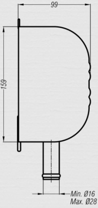
Forced - Air Convector Cebri Konvektör
